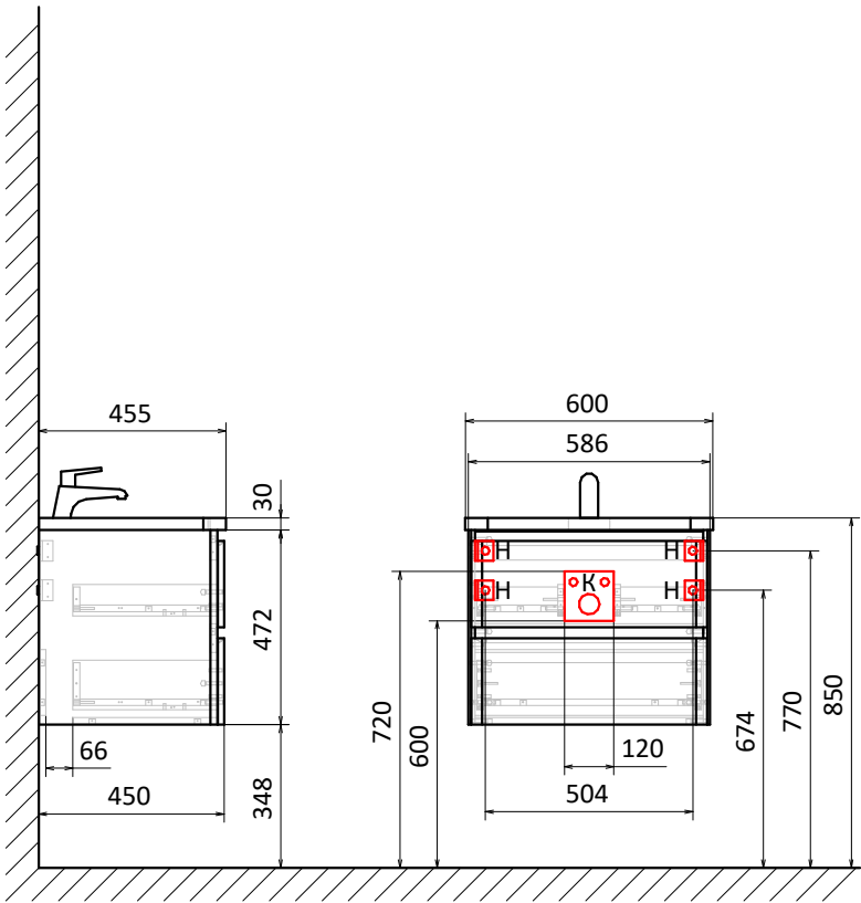
Тумба подвесная S4 60
