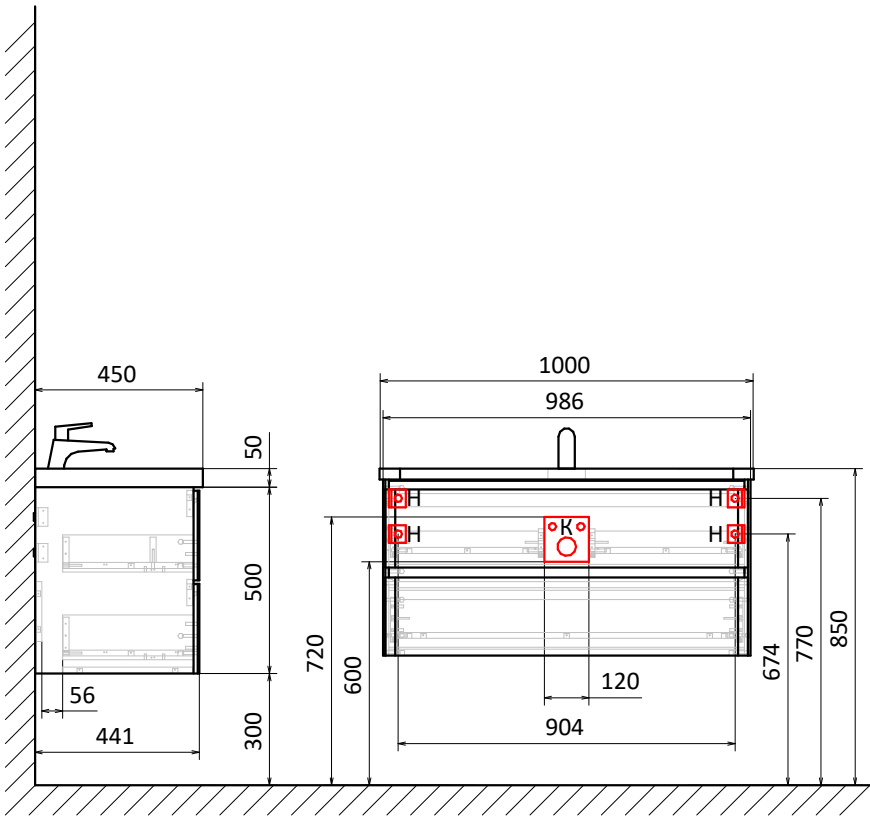
Тумба подвесная S4 100
