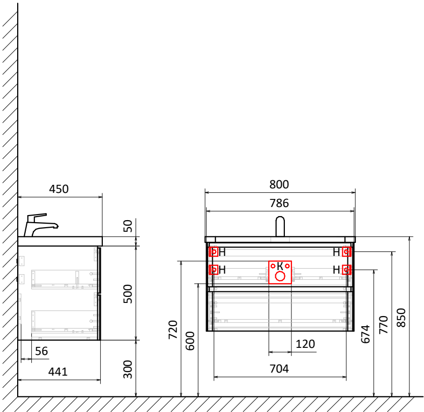
Тумба подвесная S4 80
